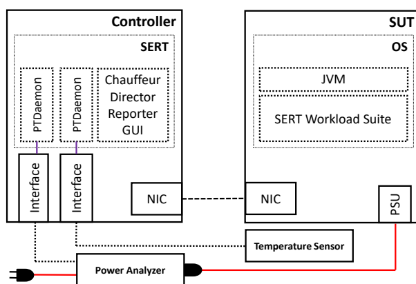
图 1: SERT 环境
